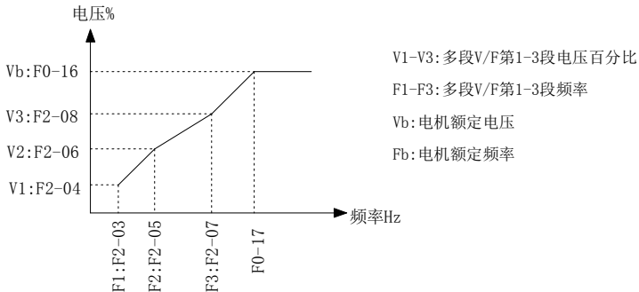
图 6-3 多点 V/F 曲线设定示意图
