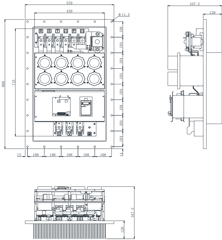
132~185kW 变频器外形图及外形尺寸示意图
