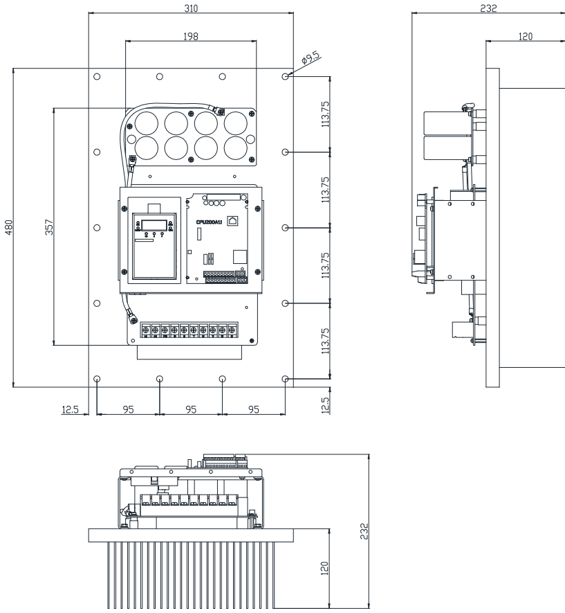
15~18.5KW 变频器外形图及外形尺寸示意图
