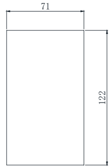
键盘托架开孔尺寸图
