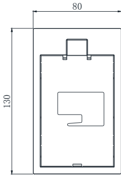
键盘托架外形尺寸图
