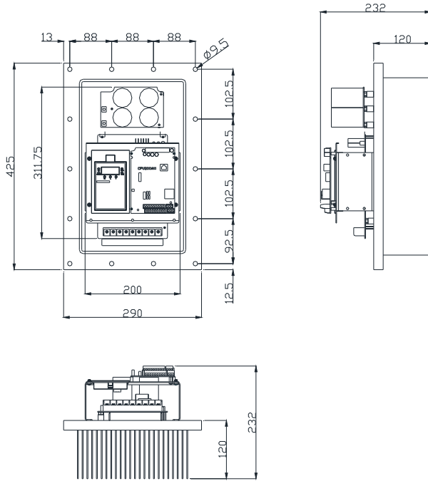
5.5~11KW(新结构)变频器外形图及外形尺寸示意图
