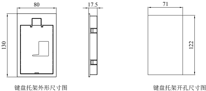
键盘托架外形尺寸图
