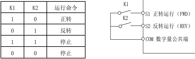
图 6-4 两线式模式 1
