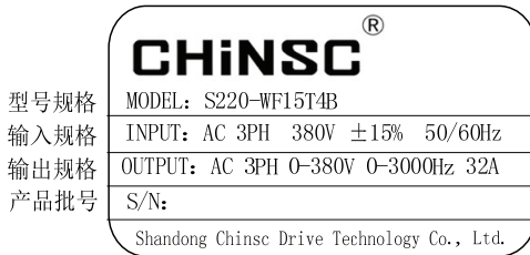
S220 系列变频器型号与技术参数
